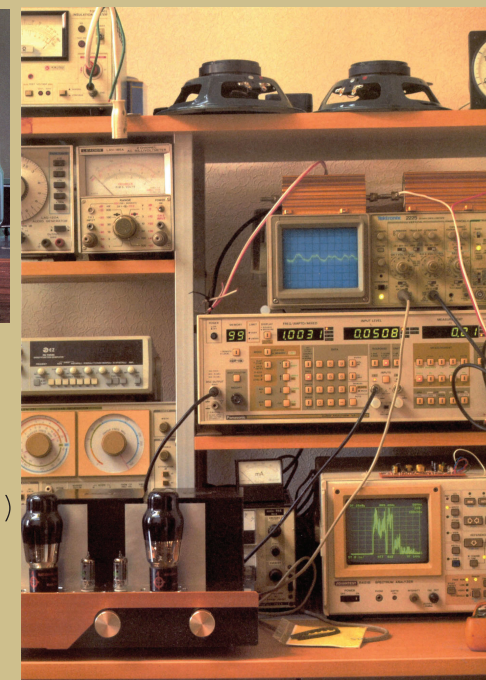
計測器(右)
